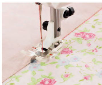
Прозрачная лапка для соединительного шва
